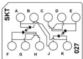
CTJ420E027 Two 66099-108 or 66139-101 ISO Cubes
