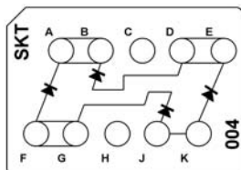
CTJ420E004 One VE08 Rectifier
