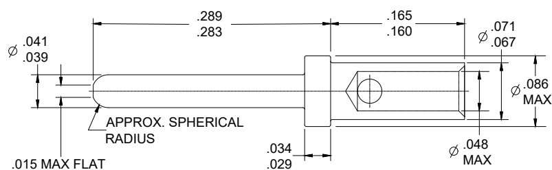
Pin - 030-9661-000
