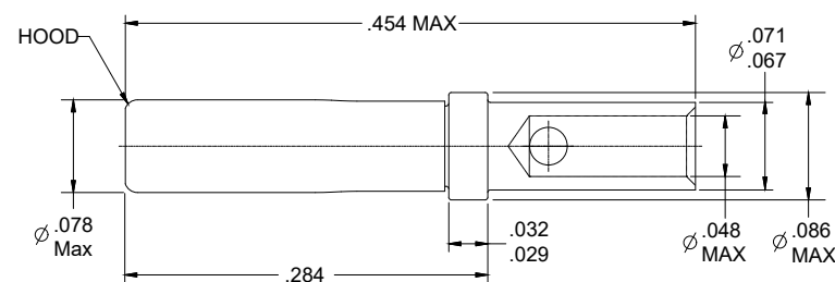
Socket - 031-9766-000
