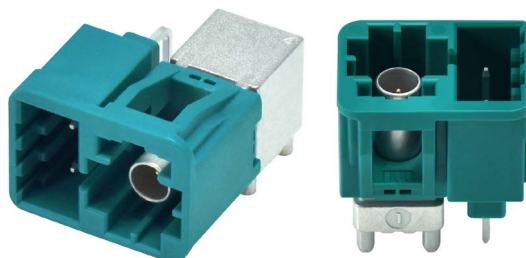
Mini FAKRA (1x1) +MQS 2Pin Right Angle and Vertical PCB Plug
