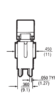
2 Pole
