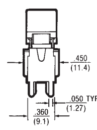
2 Pole
