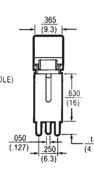
1 Pole
