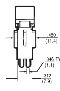
2 Pole
